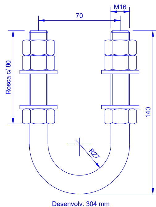
5 QZ16-140-70 (Esc 1/2)
