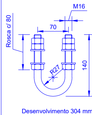
6 QZ16-140-70 (Esc 1/5)
