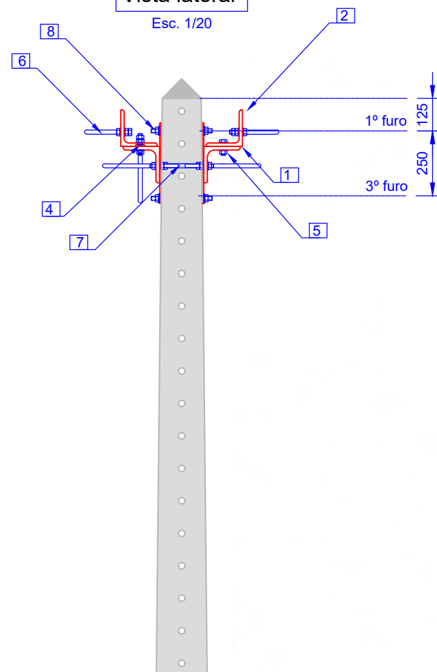
Vista lateral
