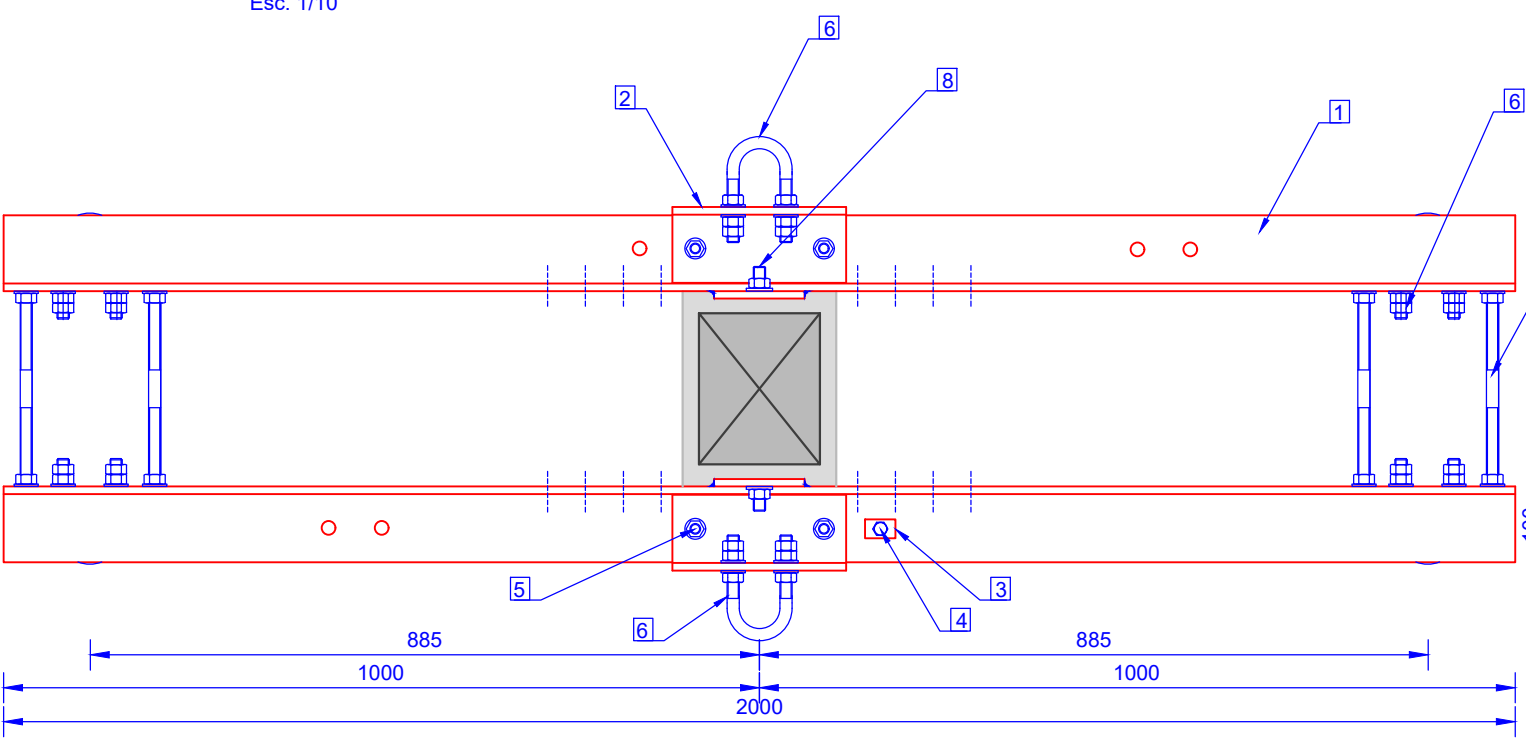
Vista superior
