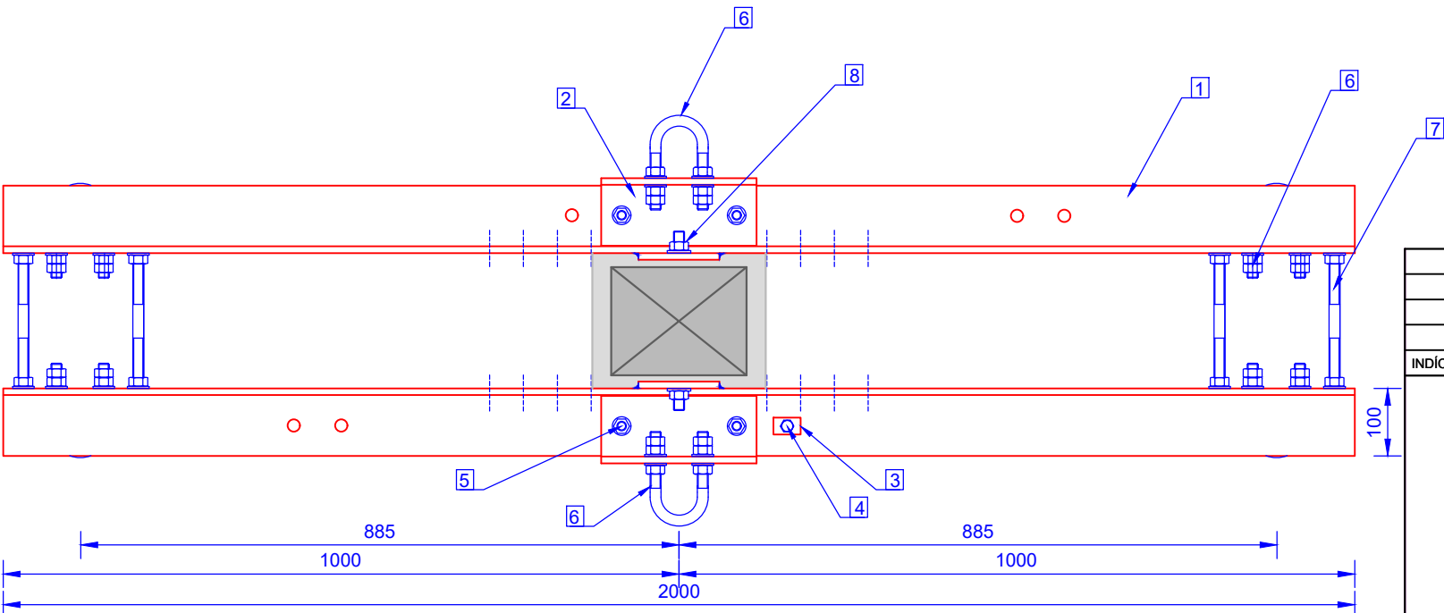
Vista superior
