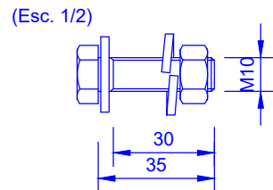
4 M10x35+P(1)+AP(1)+AM(1) (Esc. 1/2)
