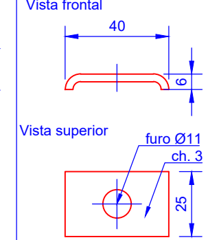
8 FLT40x25x3 (Esc 1/2)
