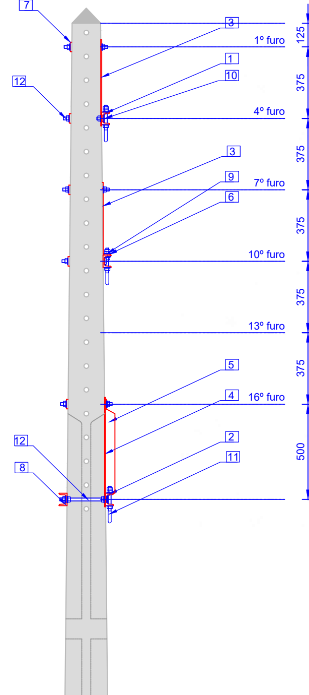
Vista lateral
