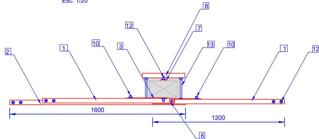
Vista superior
