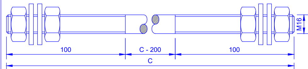
7 P16-C(100)+P(4)+AP(4) (Esc 1/2)
