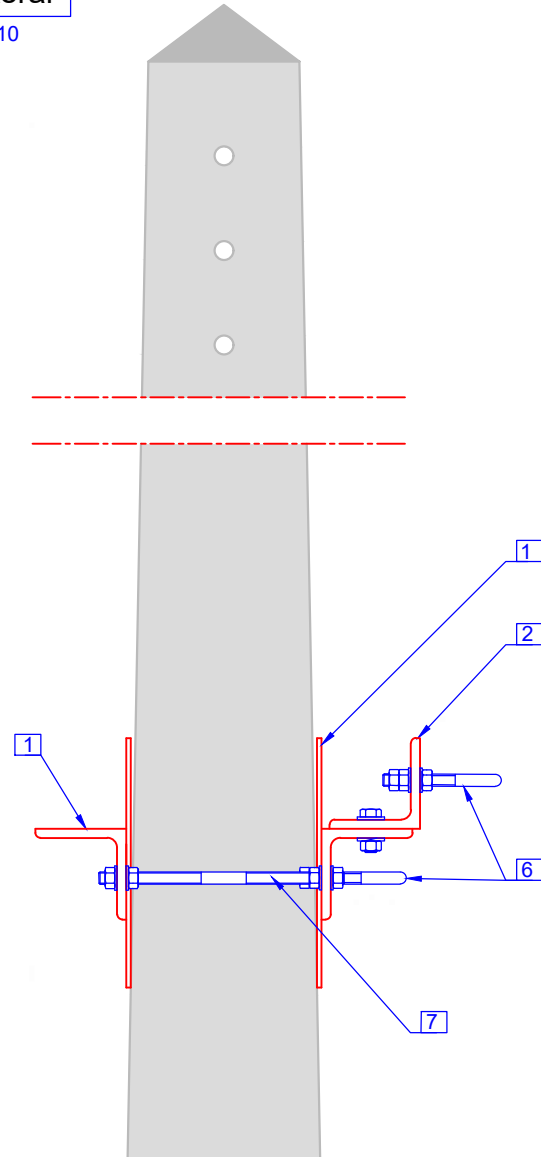
Vista lateral
