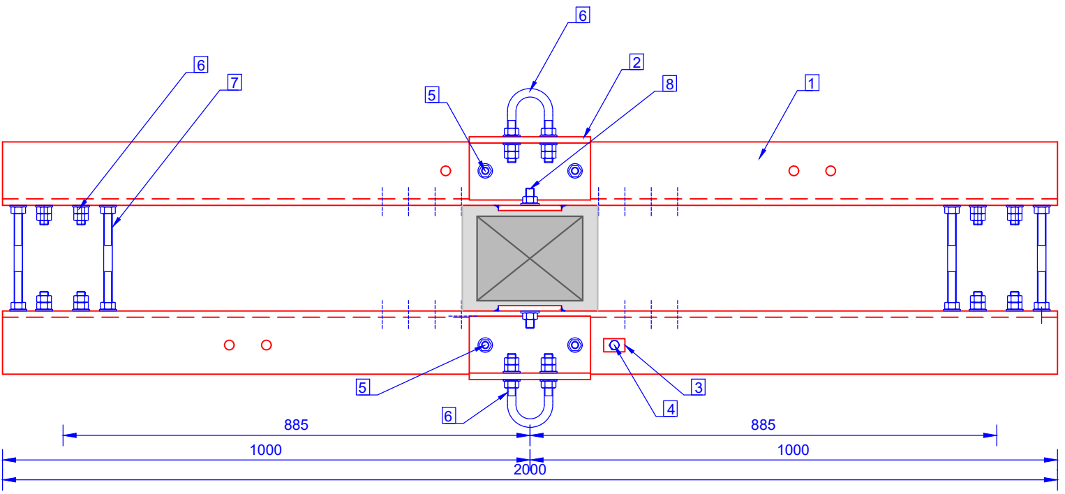
Vista superior
