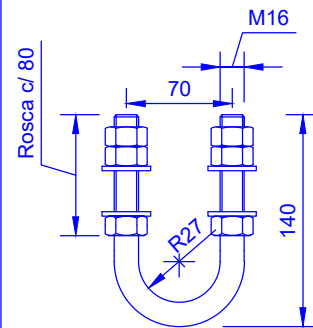
6 QZ16-140-70 (Esc 1/5)
