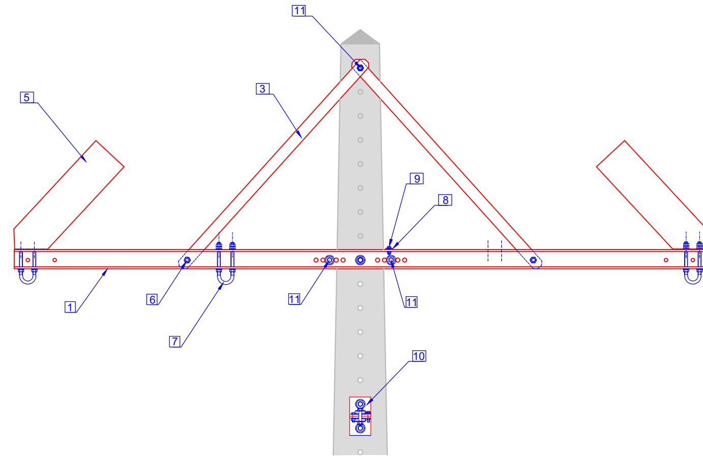
Vista frontal Esc. 1/20
