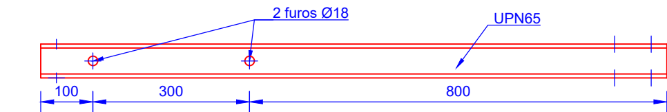
1 UPN65 (Esc 1/10)
