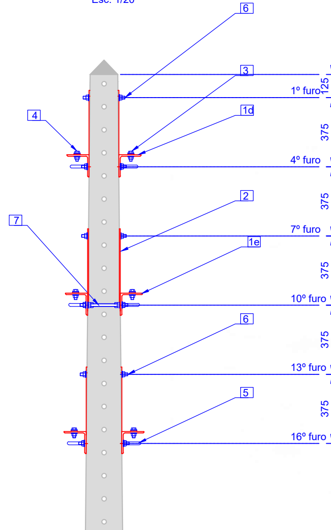
Vista lateral
