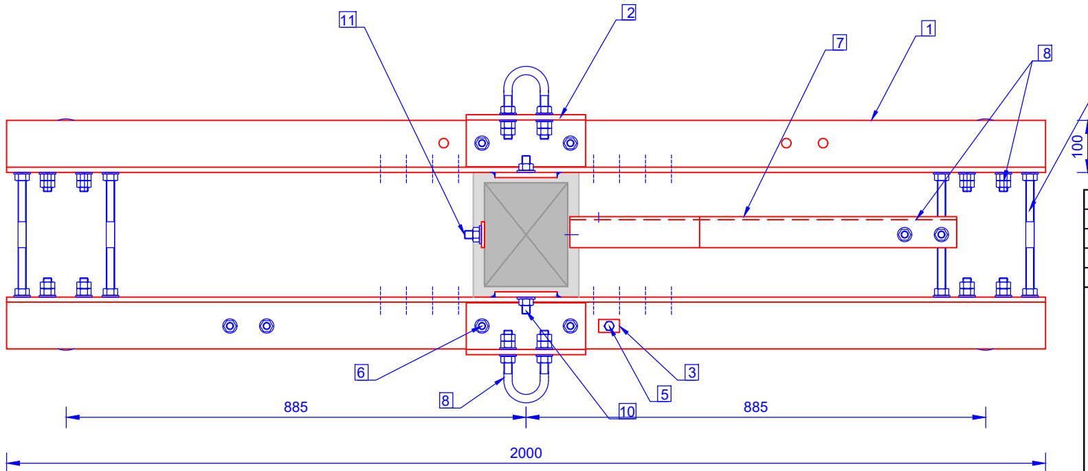
Vista superior
