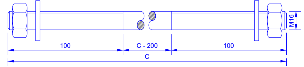
8 9 P16-C(100)+P(2)+AP(2) (Esc. 1/2)
