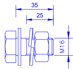
12 M16x35x25+P(1)+AP(1)AM(1) (Esc. 1/2)
