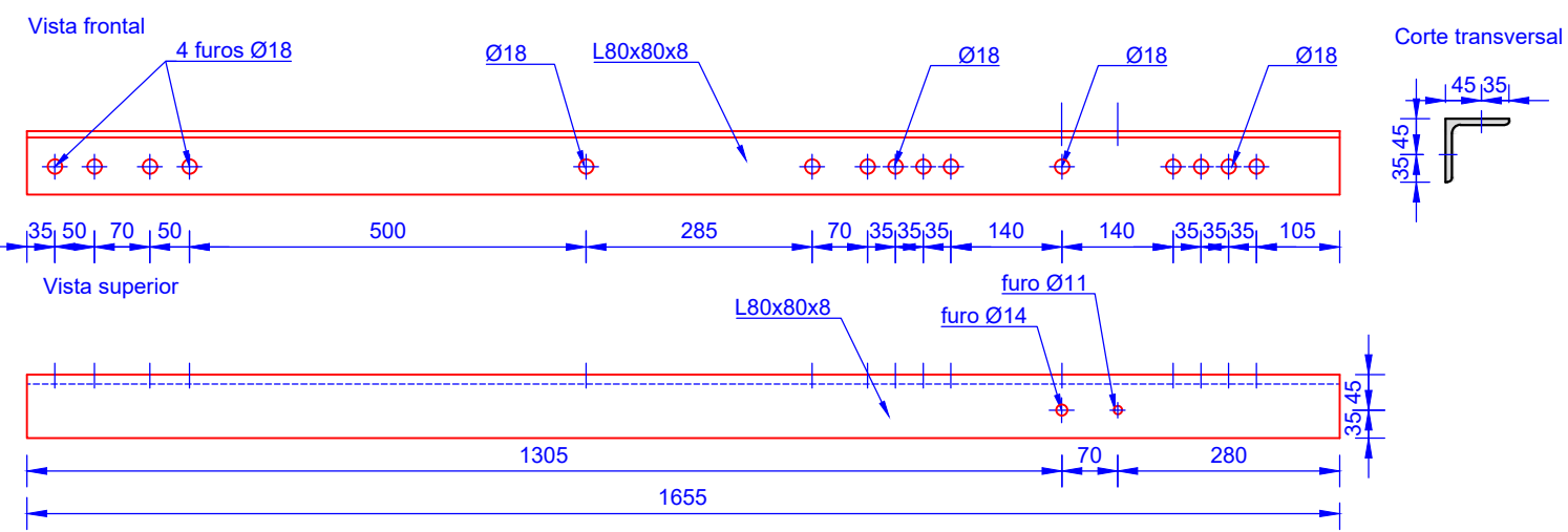
5 QZ16-140-70 (Esc 1/2)
