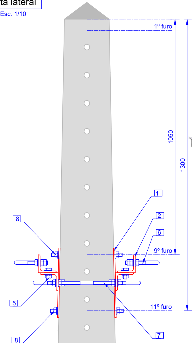
Vista lateral
