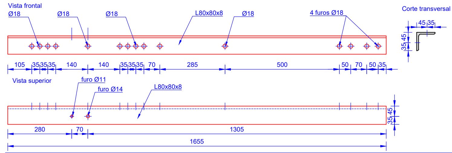
1e L80x80x8 (Esc 1/10)
