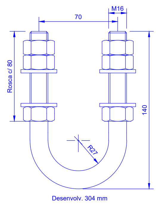
5 QZ16-140-70 (Esc 1/2)
