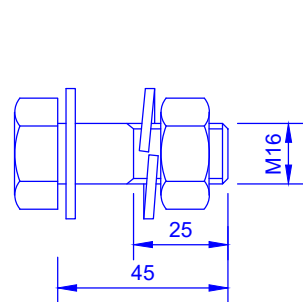
5 M16x45x25+P(1)+AP(1)+AM(1) (Esc. 1/2)
