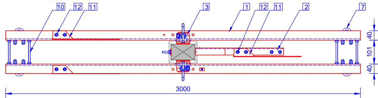
Vista superior
