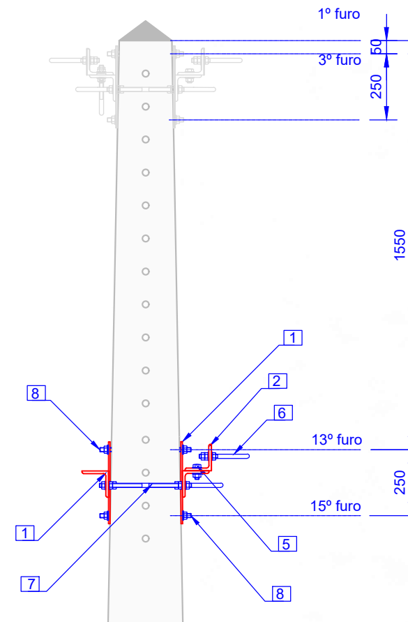
Vista lateral
