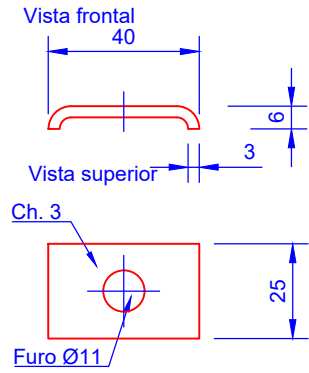
4 FLT40x25x3 (Esc. 1/2)
