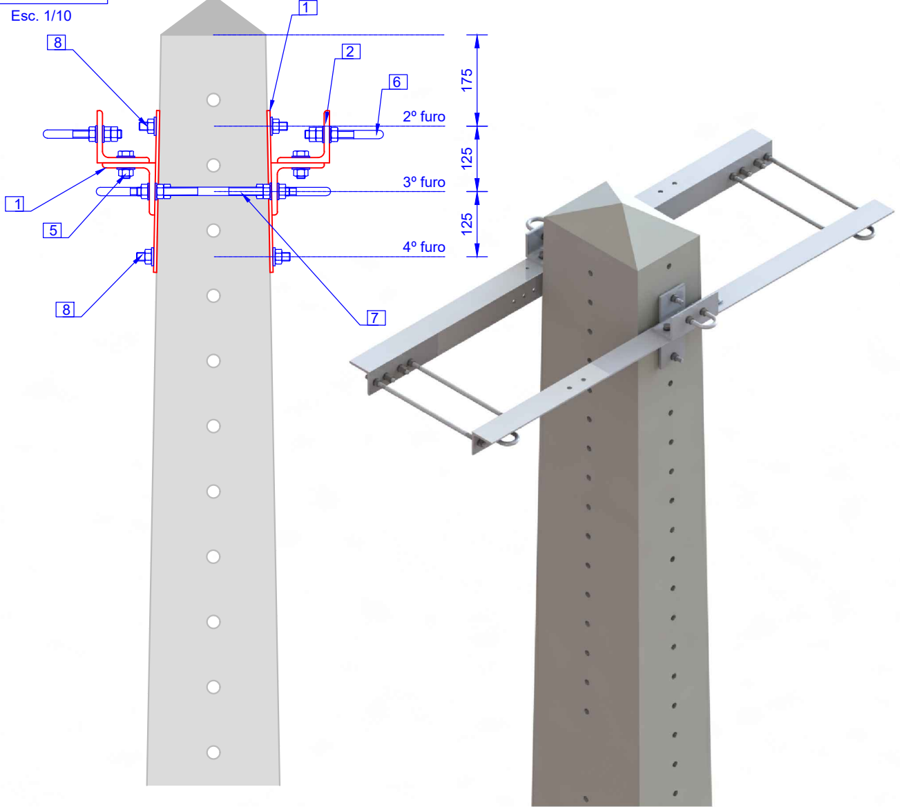
Vista lateral
