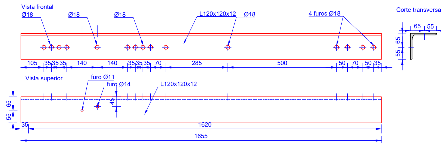
2e L120x120x12 (Esc 1/10)
