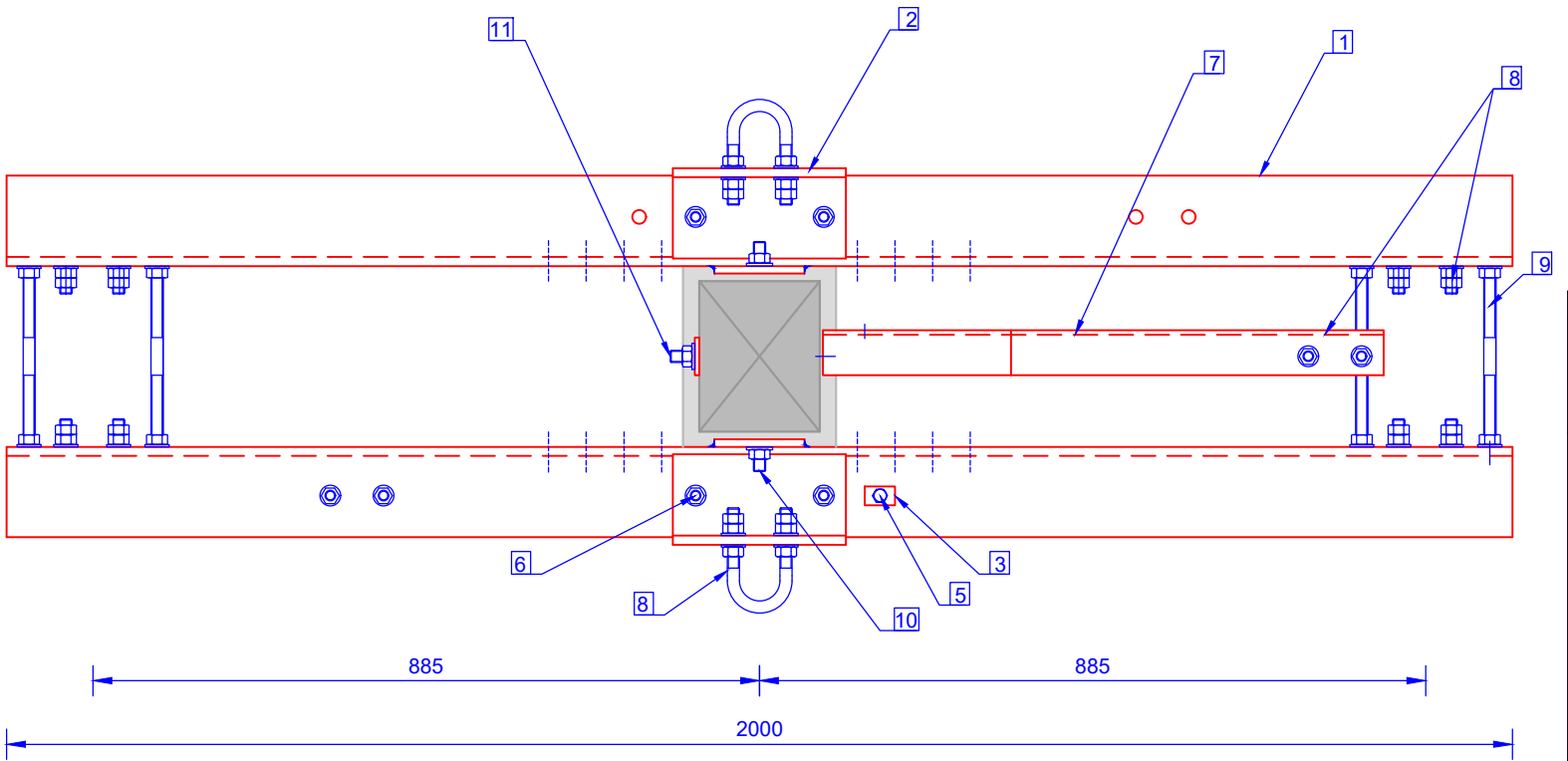
Vista superior
