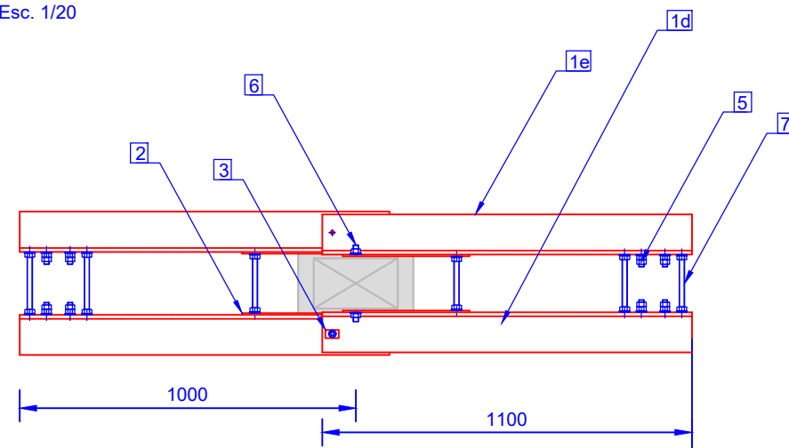
Vista superior
