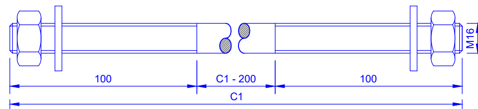
8 P16-C(100)+P(2)+AP(2) (Esc 1/2)
