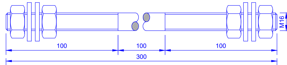
13 P16-300(100)+P(4)+AP(4) (Esc 1/2)
