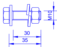
4 M10x35+P(1)+AP(1)+AM(1) (Esc. 1/2)
