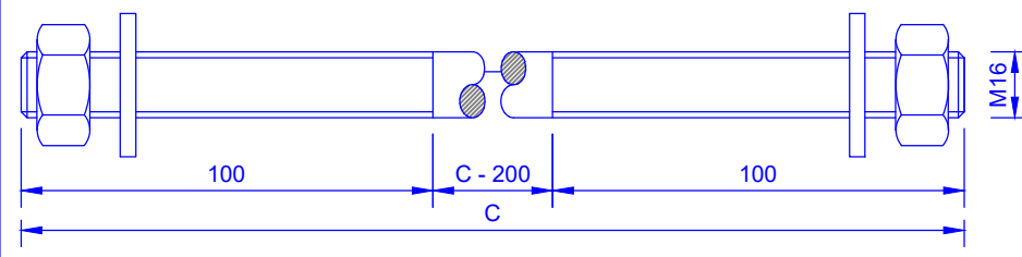
6 P16-C(100)+P(2)+AP(2) (Esc 1/2)
