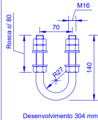
6 QZ16-140-70 (Esc 1/5)
