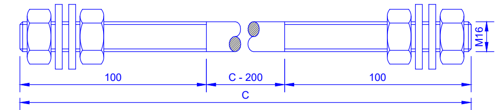
7 P16-C(100)+P(4)+AP(4) (Esc 1/2)
