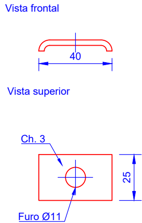
2 FLT40x25x3 (Esc. 1/2)
