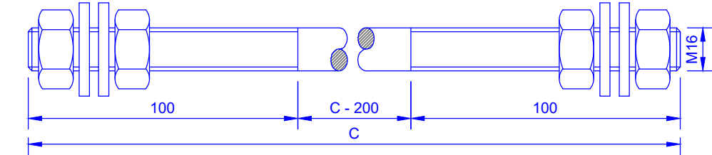
10 P16-C(100)+P(4)+AP(4) (Esc. 1/2)
