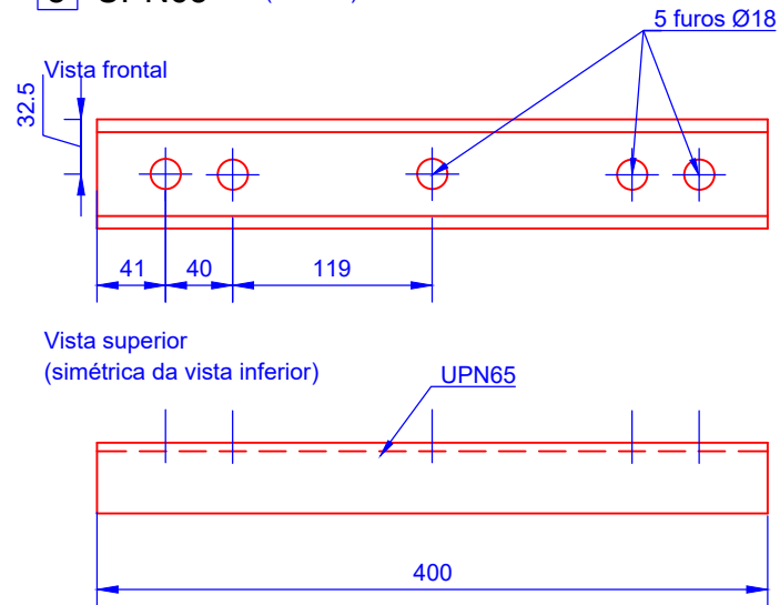
8 UPN65 (Esc 1/5)
