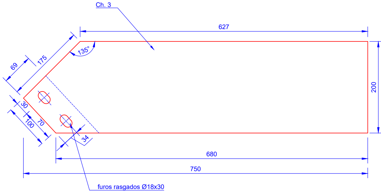
11 CH3 (Esc. 1/5)
