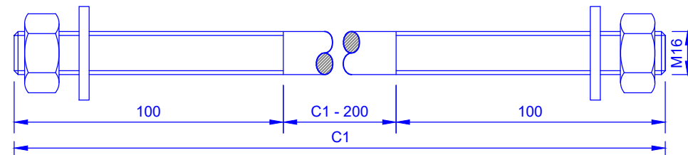
8 P16-C1(100)+P(2)+AP(2) (Esc 1/2)
