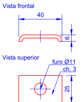
8 FLT40x25x3 (Esc 1/2)
