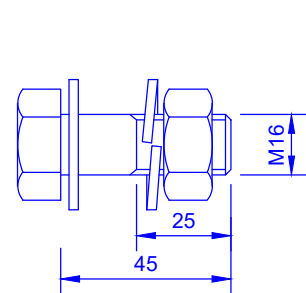
5 M16x45x25+P(1)+AP(1)+AM(1) (Esc. 1/2)
