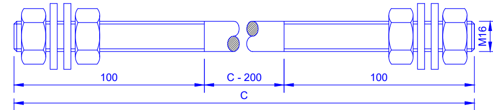
7 P16-C(100)+P(4)+AP(4) (Esc 1/2)
