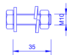
6 M10x35+P(1)+AP(1)+AM(1) (Esc. 1/2)
