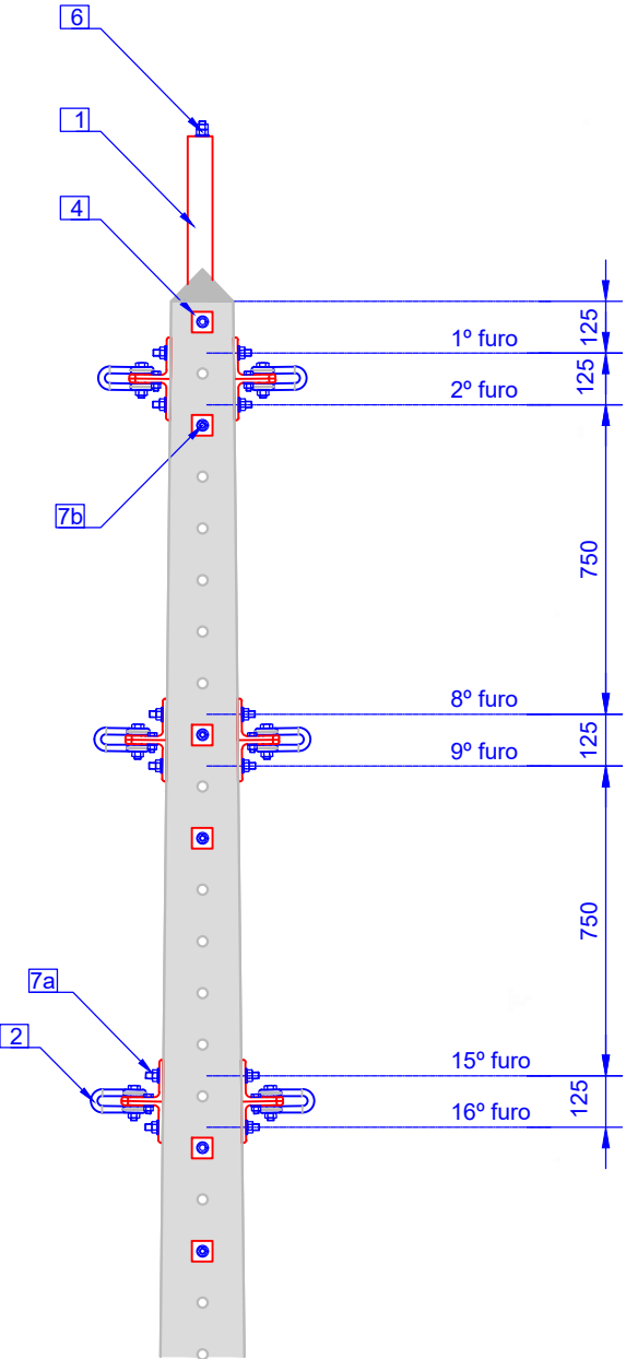
Vista lateral
