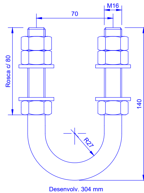
5 QZ16-140-70 (Esc 1/2)
