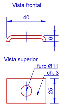
6 FLT40x25x3 (Esc 1/2)
