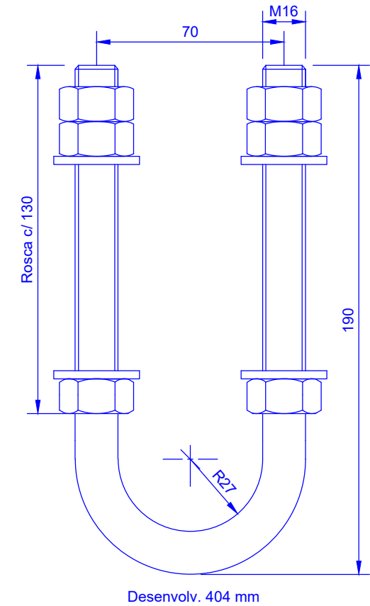
7 QZ16-190-70 (Esc 1/2)
