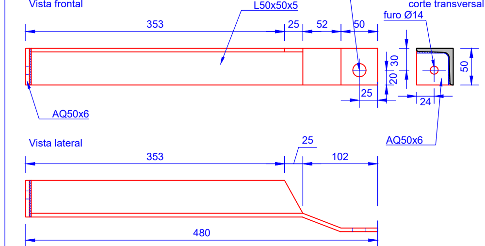
7 P16-C(100)+P(4)+AP(4) (Esc 1/2)
