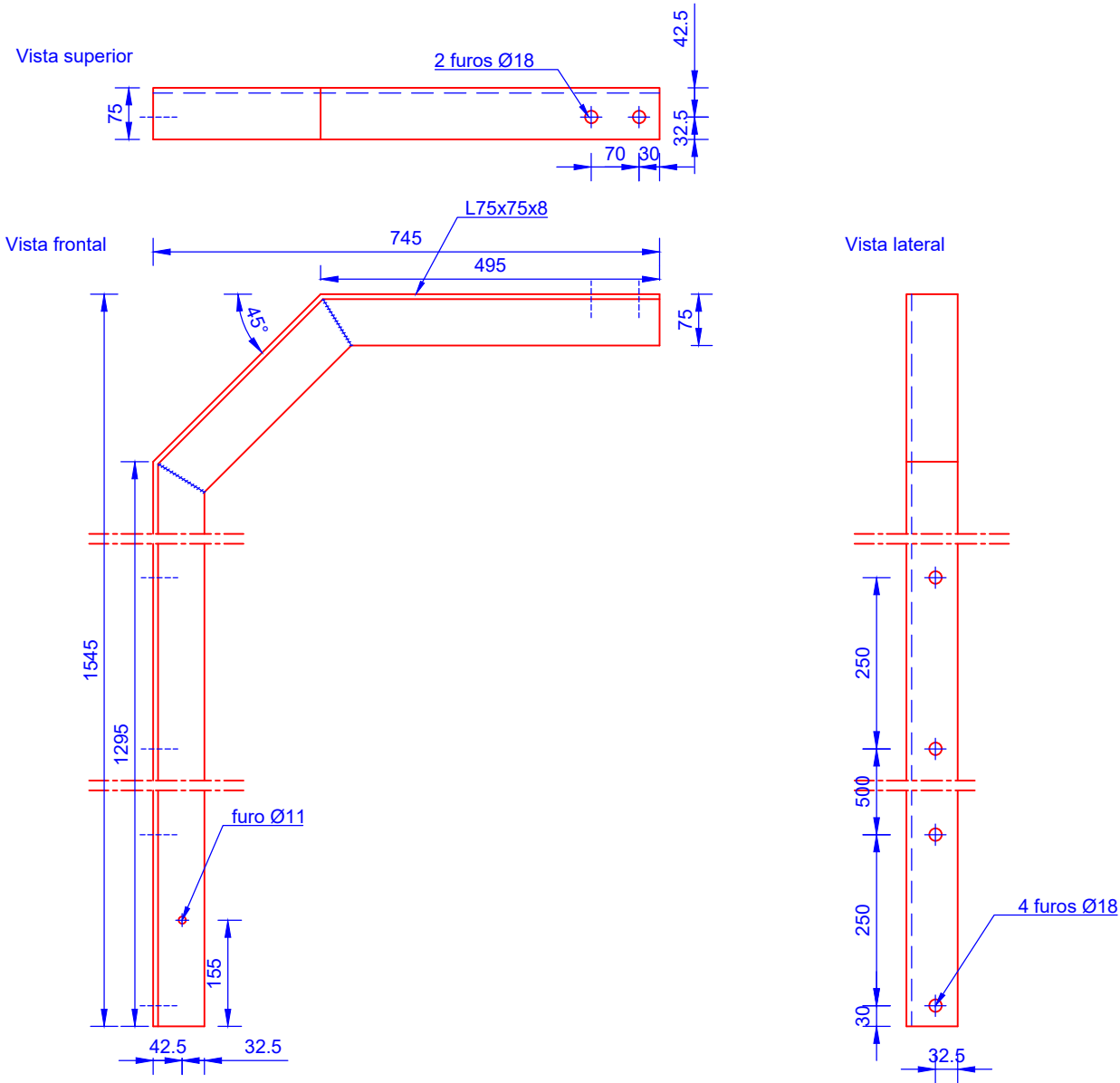
1 L75x75x8 (Esc. 1/10)
