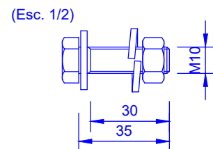
4 M10x35+P(1)+AP(1)+AM(1)
