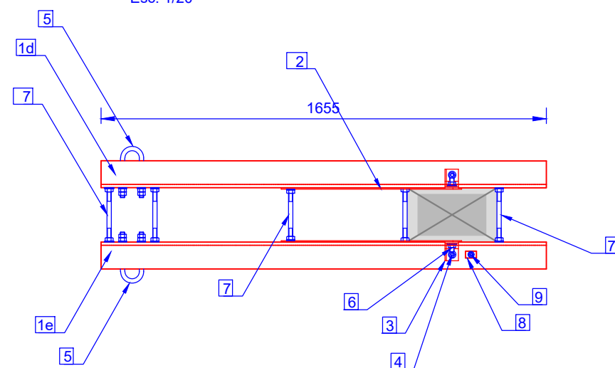
Vista superior
