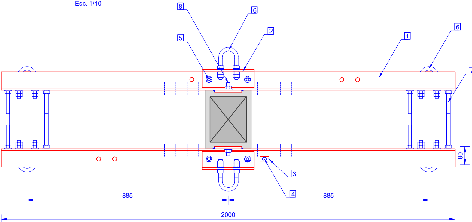
Vista superior
