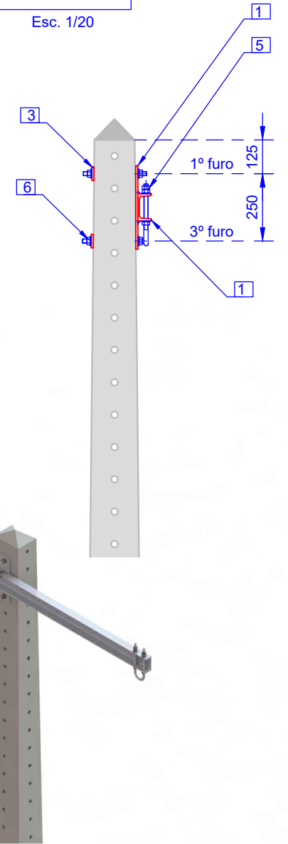
Vista lateral
