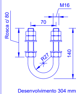
6 QZ16-140-70 (Esc 1/5)
