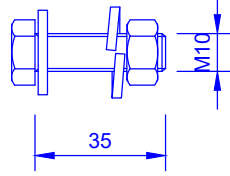
6 M10x35+P(1)+AP(1)+AM(1) (Esc. 1/2)
