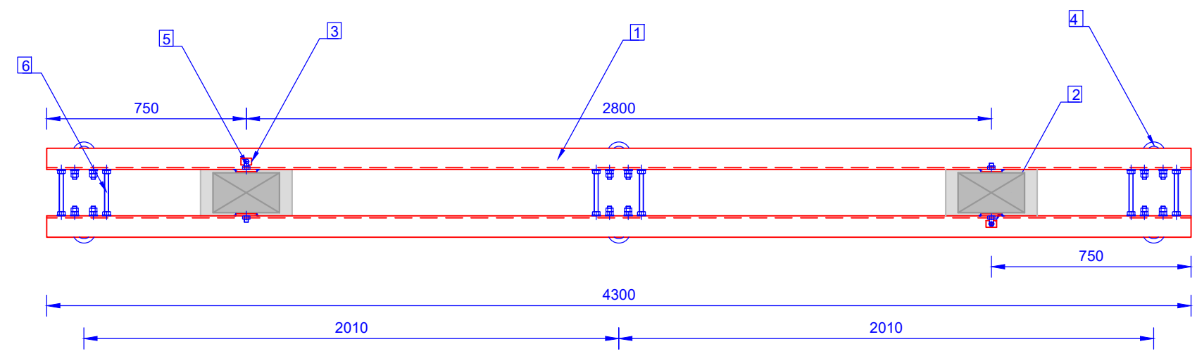
Vista superior
