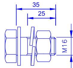
5 M16x35x25+P(1)+AP(1)+AM(1) (Esc. 1/2)
