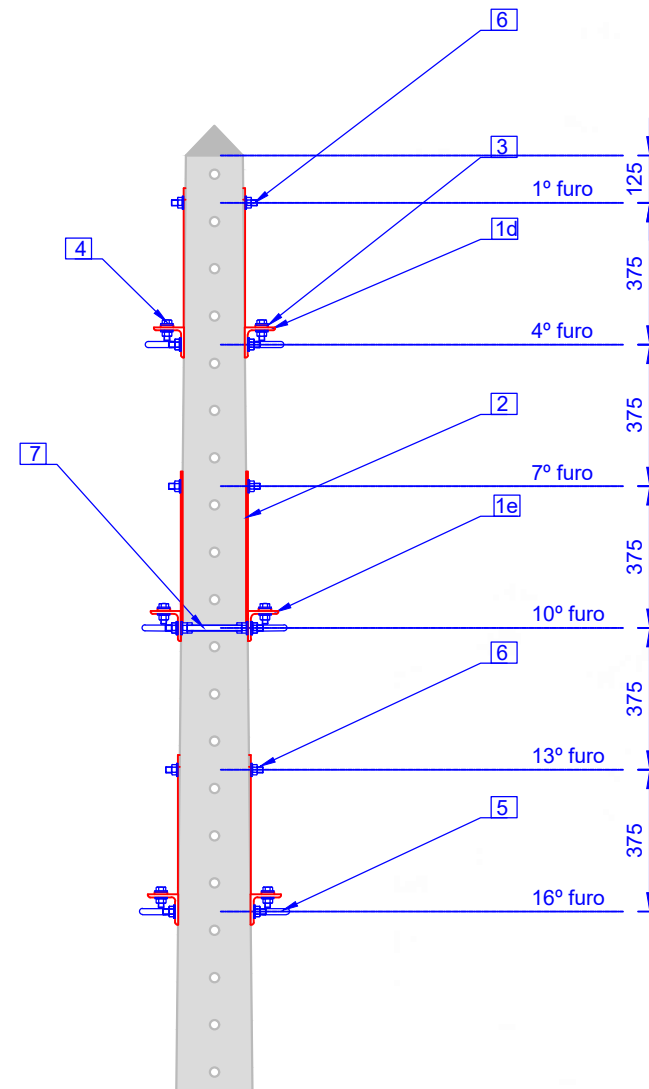
Vista lateral
