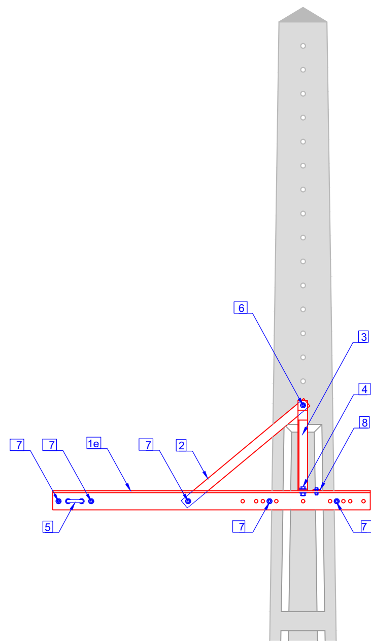
Vista superior
