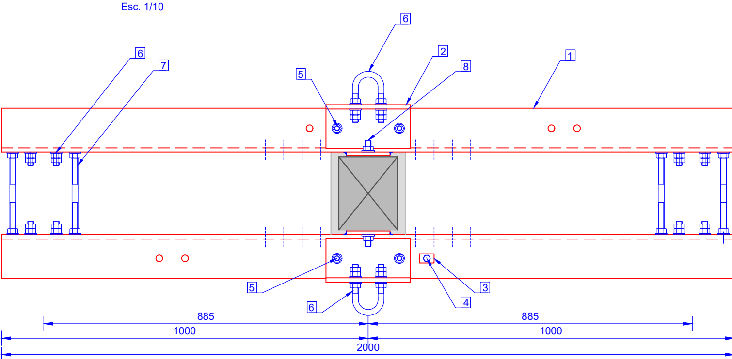
Vista superior
