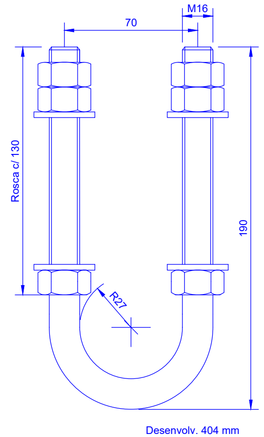
11 QZ16-190-70 (Esc. 1/2)
