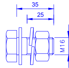
10 M16x35x25+P(1)+AP(1)AM(1) (Esc. 1/2)
