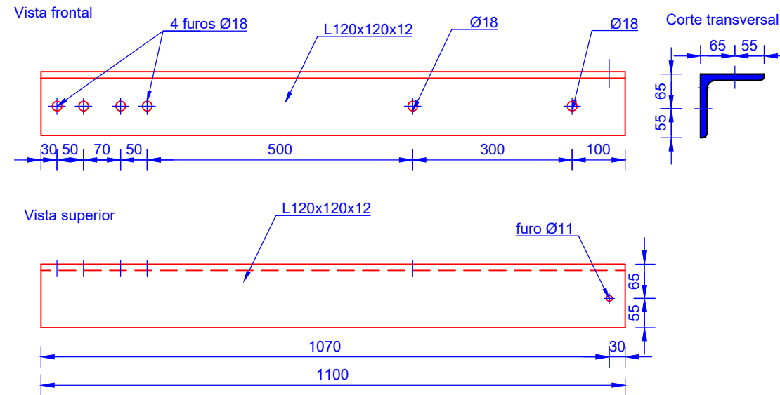
1e L120x120x12 (Esc 1/10)
