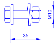
3 M10x35+P(1)+AP(1)+AM(1) (Esc. 1/2)
