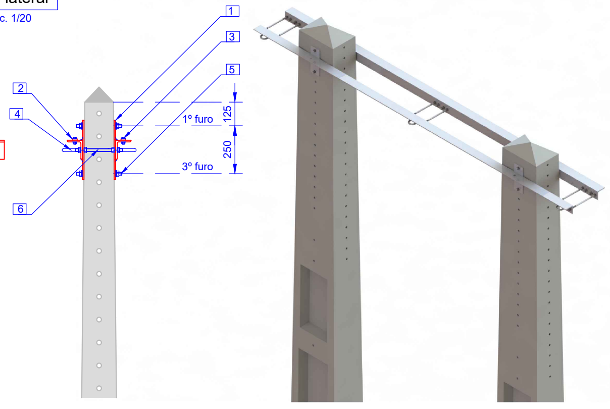
Vista lateral
