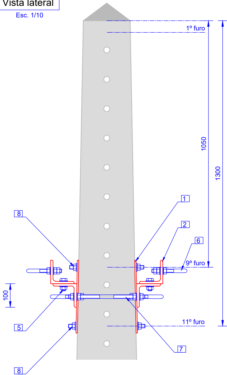
Vista lateral
