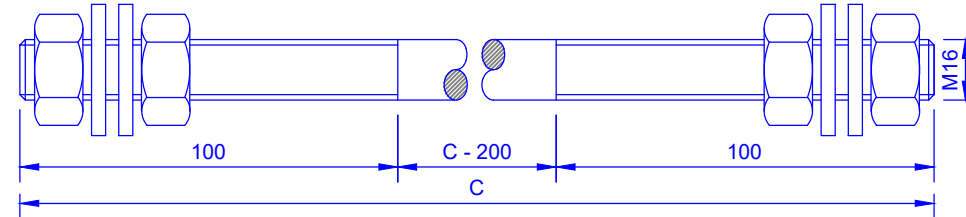
7 P16-C(100)+P(4)+AP(4) (Esc 1/2)
