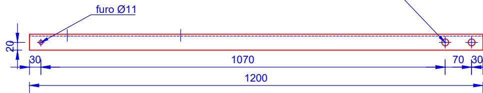
3 FLT40x25x3 (Esc 1/2)
