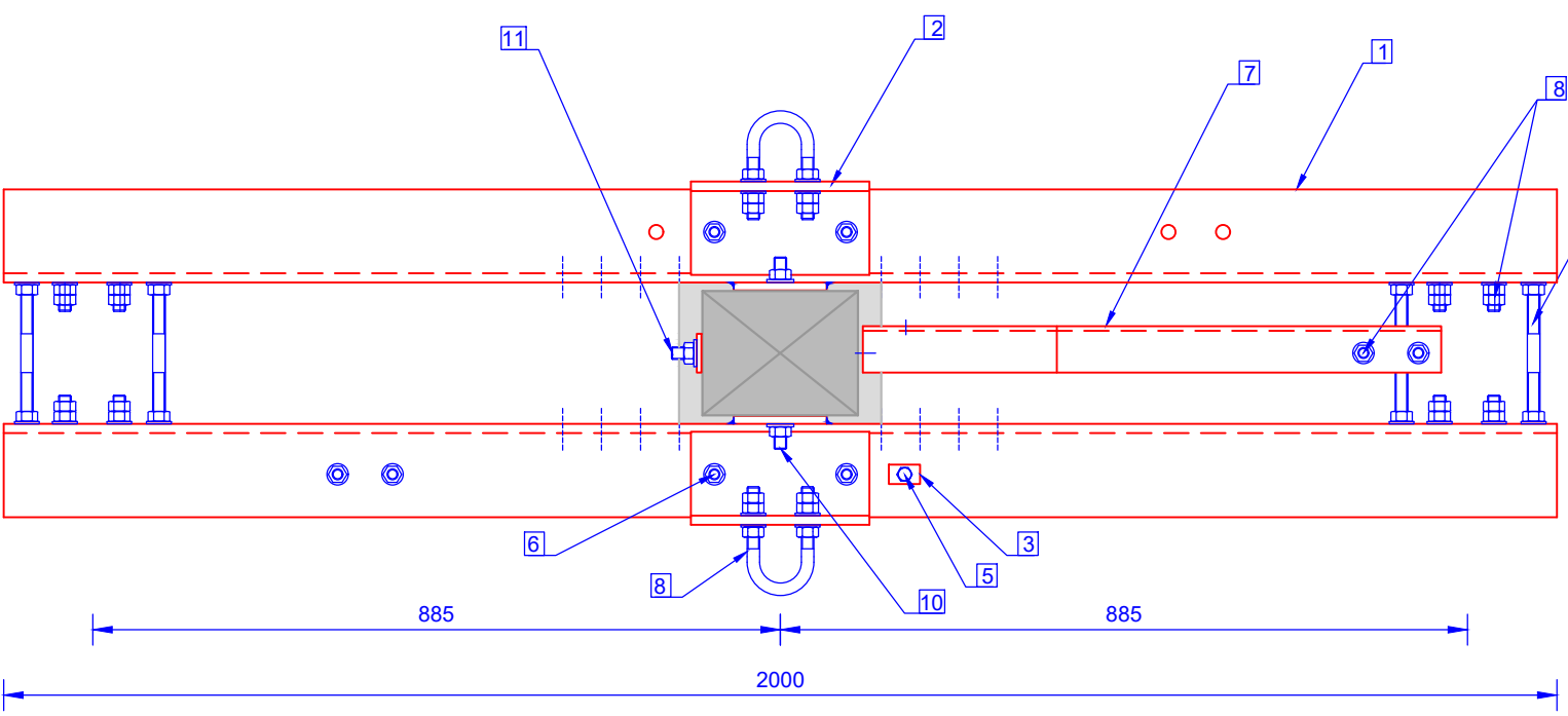
Vista superior
