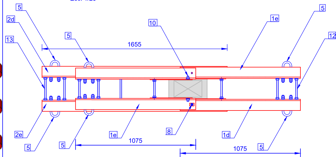
Vista superior
