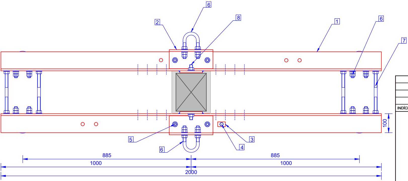
Vista superior
