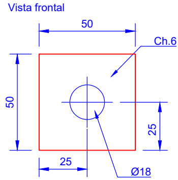
5 AQ50x6 (Esc. 1/2)
