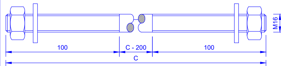
6 P16-C(100)+P(2)+AP(2) (Esc 1/2)
